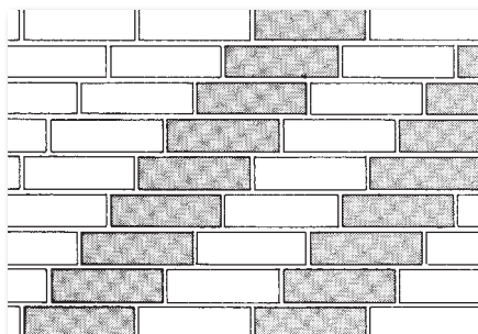
Ложковая перевязка со сдвигом на кирпичи по диагонали
