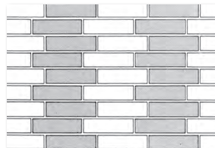
Ложковая перевязка со сдвигом на кирпичи по вертикали
