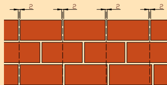
Несовпадение вертикальных швов
