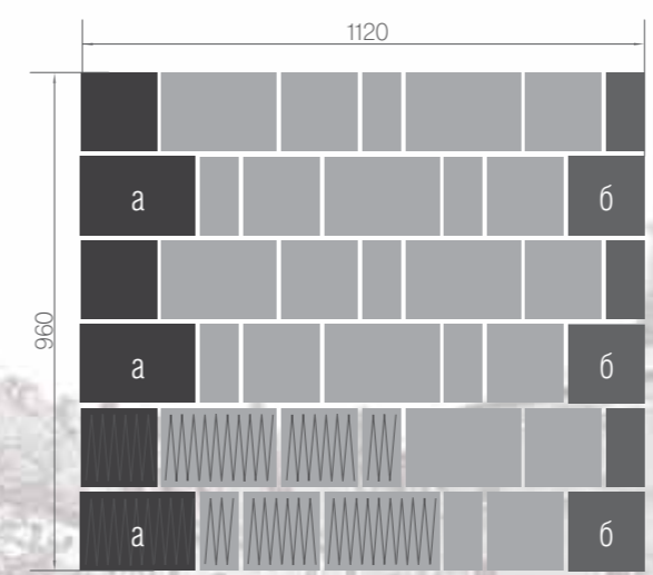
1 Вид плитки на поддоне
