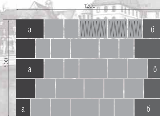
1 Вид плитки на поддоне
