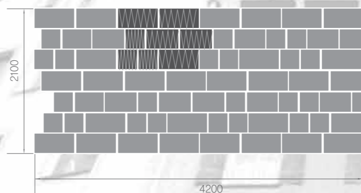
Вид площади при укладке элемента №2
