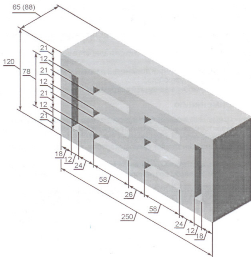
Рисунок А.1.3 — Кирпич формата 1(1,4) НФ с восемью щелевидными пустотами
