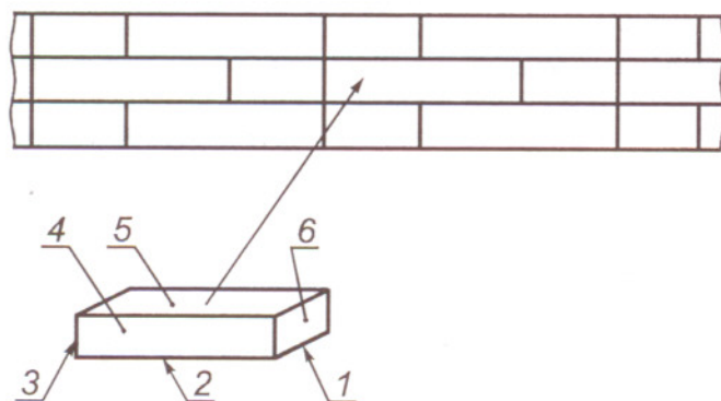
1 — ширина; 2 — длина; 3 — толщина; 4 — ложок; 5 — постель; 6 — тычок
