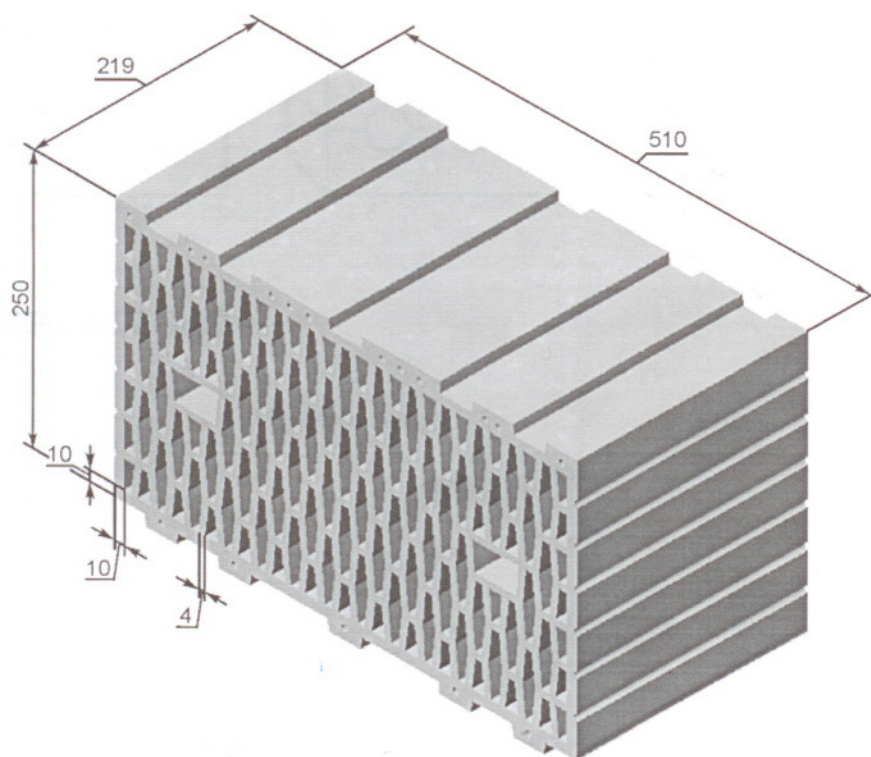
Рисунок А.1.23 — Камень крупноформатный 14,3 НФ
