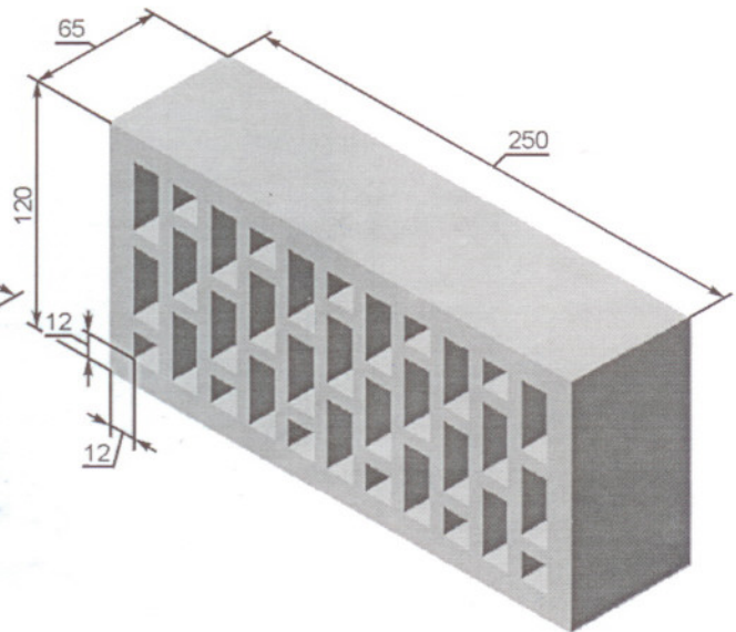
Рисунок А.1.10 — Кирпич формата 1 НФ с 33 пустотами
