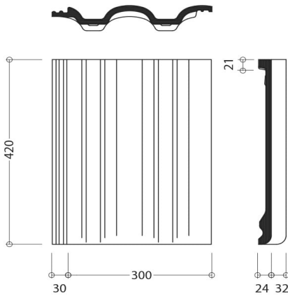
Цементно-песчаная черепица Таунус
