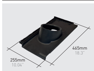
Q118*K | Innova/Vienna chimney roof tile klinker
