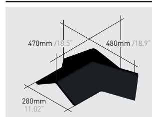
Q111*K | Atica 120o 3 way ridge klinker
